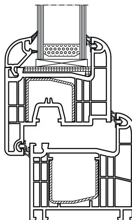
CORTE B - B
